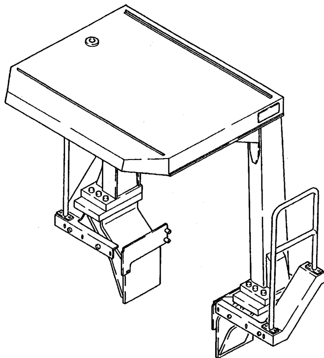
ROPS CANOPY ロプス
