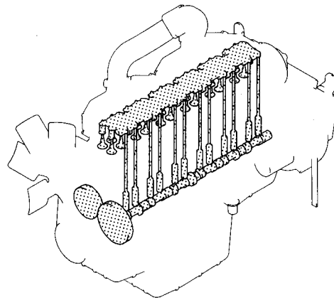
VALVE MECHANISM バルブ メカニズム
