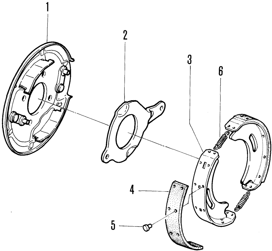
トランスミッション パーキング ブレーキ Fig. 24 TRANSMISSION PARKING BRAKE
