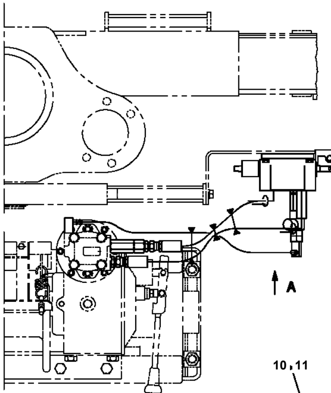
(4連弁時リヤジャッキ、セルフウインチ、サービスポート)
