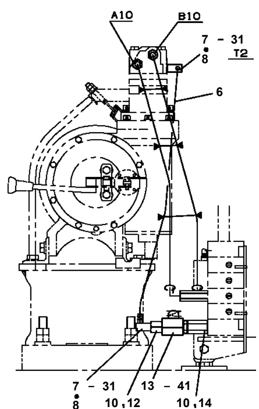
(2連弁時セルフウインチ、サービスポート)
