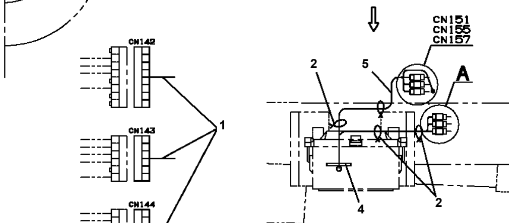
A キャブ後方第一クロスメンバ部
