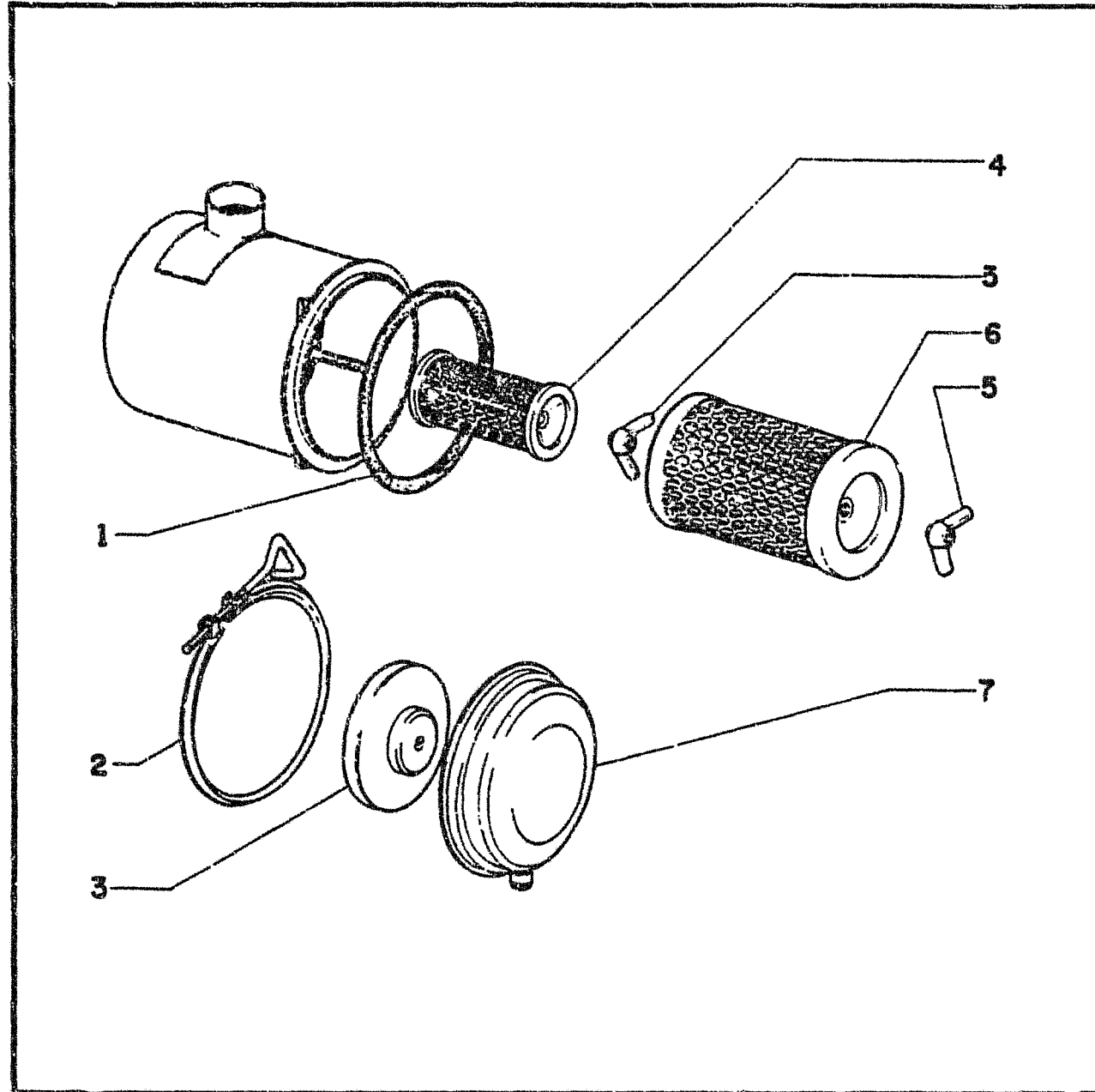
AIR CLEANER FILTRO DE AR A2.23 1
