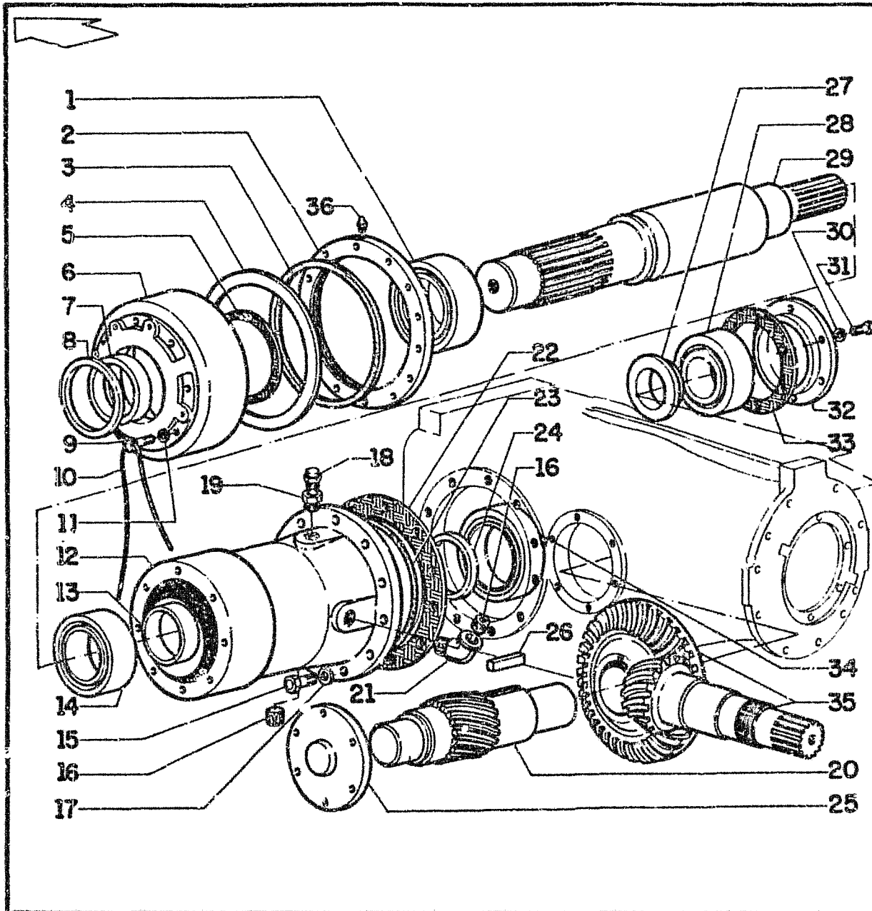
REAR AXLE EIXO TRASEIRO
