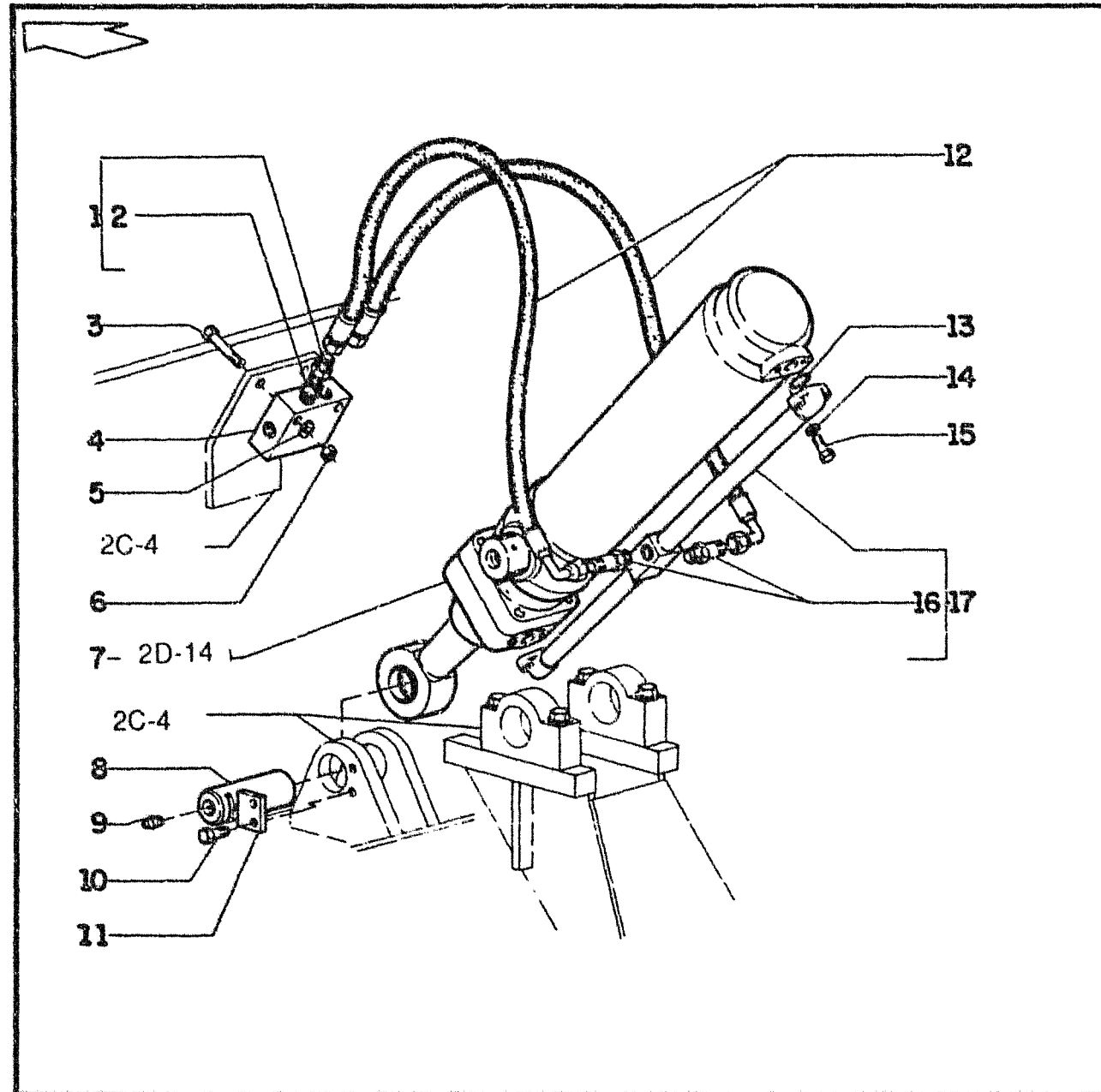
RIPPER PIPING CYLINDER TUBULAÇÃO DO RIPPER E CILINDRO
