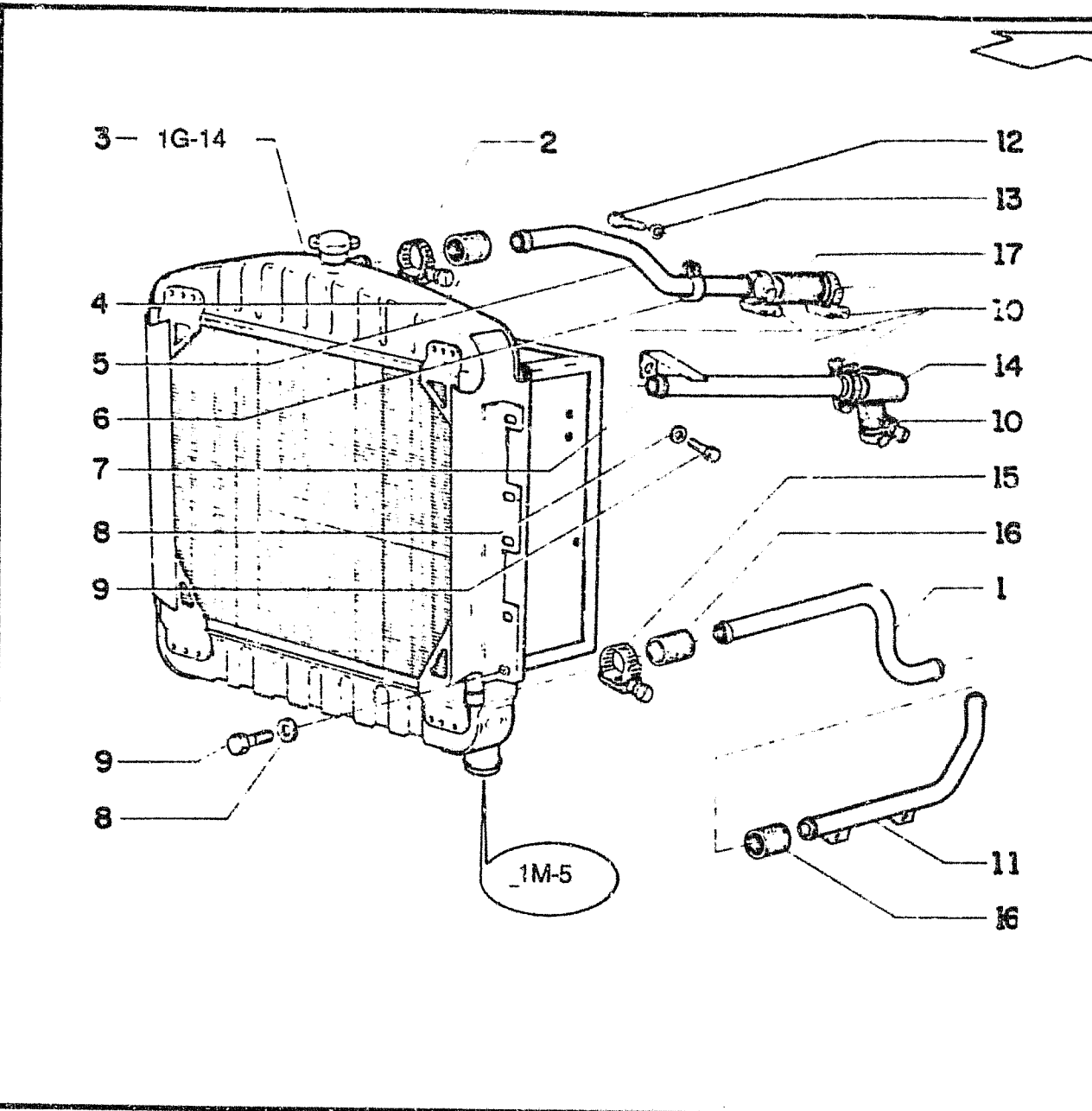
RADIATOR & PIPING RADIADOR E TUBULAÇÕES
