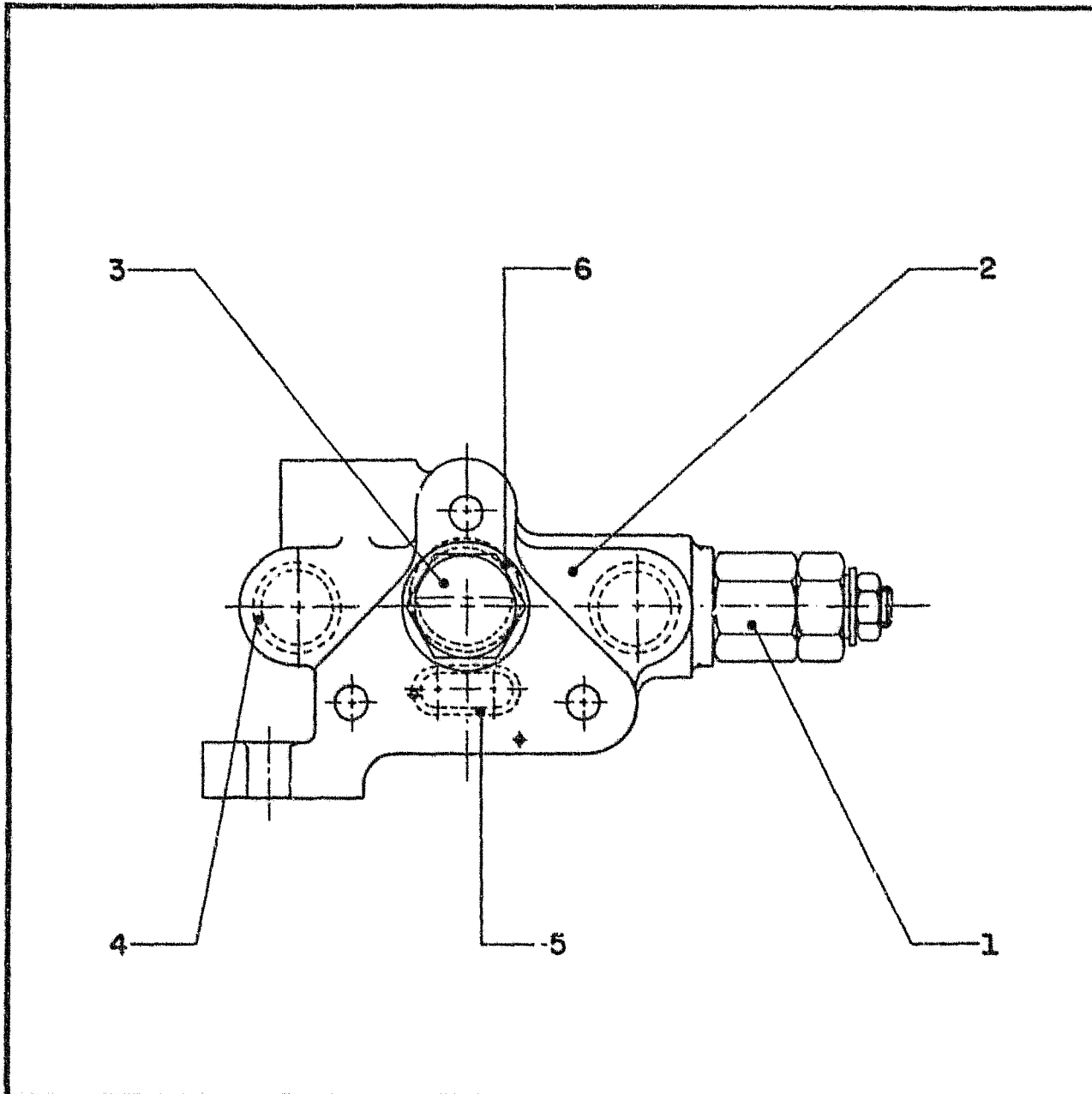
VALVE ASSEMBLY LEFT MAIN RELIEF VALVE CONJUNTO DA VALVULA ESQUERDO
