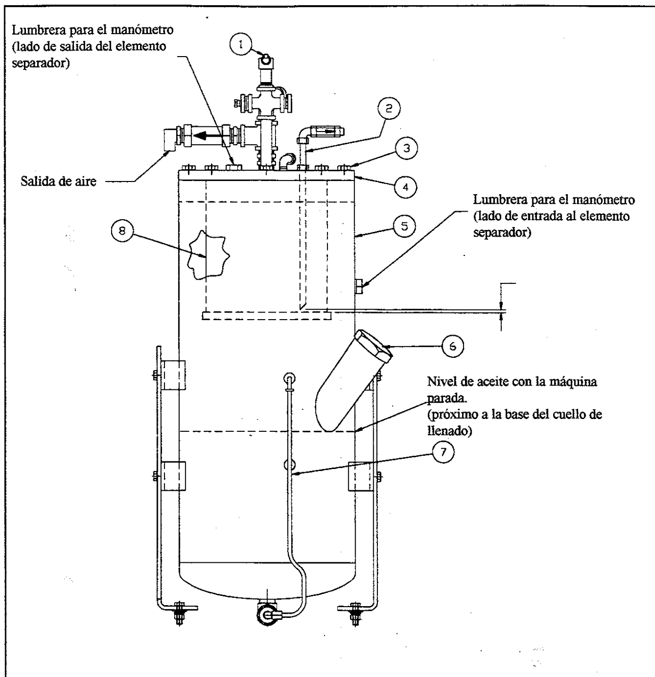
Fig. 5-1 Depósito receptor de aire
